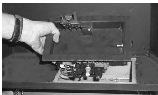
Schéma 3 : Soulever le dispositif du plateau de la valve de la valve
