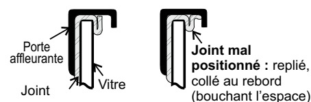
Position correcte de la porte, de la vitre et du joint.
